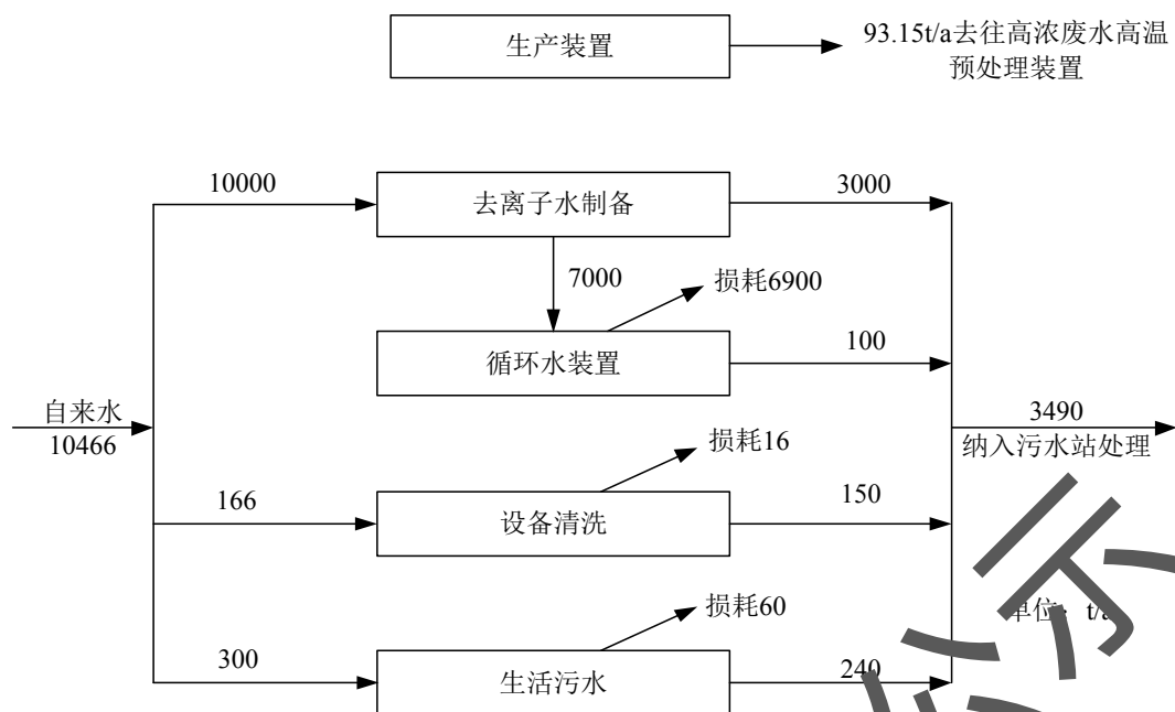
图 4.4-1 本项目水平衡图
