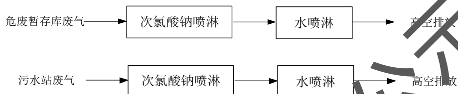
图 7.1-2 本项目污水站、危废暂存库废气处理工艺
