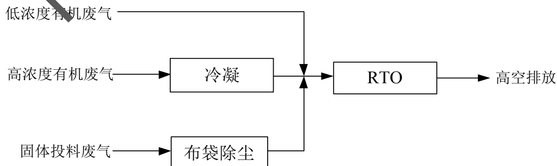
图 7.1-1 本项目工艺废气处理工艺
